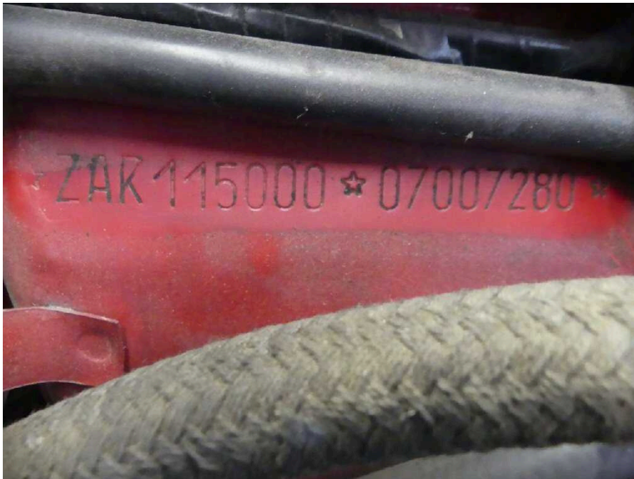
Bild 5: VIN, Fahrgestellnummer
